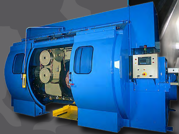
Görgős sodró: valós egyréteg
