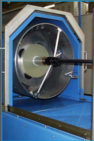
Taping (szalagtekercselés): koncentrikus & hosszanti
